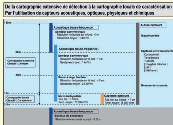
Figure 3 : liste des outils de cartographie et de mesure implantés sur les AUV déployables jusqu'à ~ 6.000 mètres.
